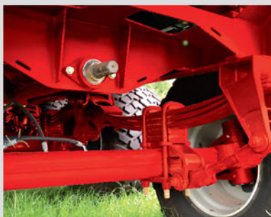
EJES DIRECCIONALES CON BLOQUEO. CHASIS AKRON.
