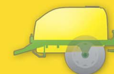
Eje fijo: 12,4 x R36 12,4 x R46 Trocha: 1,4 - 2,10 mts
